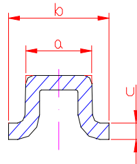
Profilquerschnitt Wellrohr Profil Section Tubing
