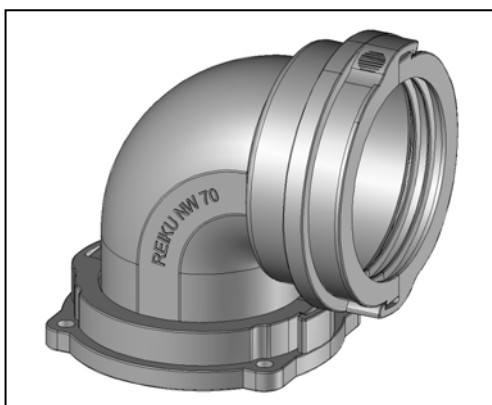
Drehbarer 90° Winkelanschluss 90° Swivelling Elbow NW70: PASOB/G-70
